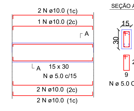
VIGAS (15X30) - CAIXA D'ÁGUA
