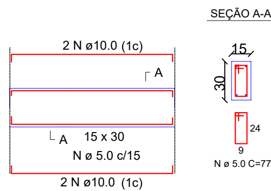
VIGAS (15X30)
