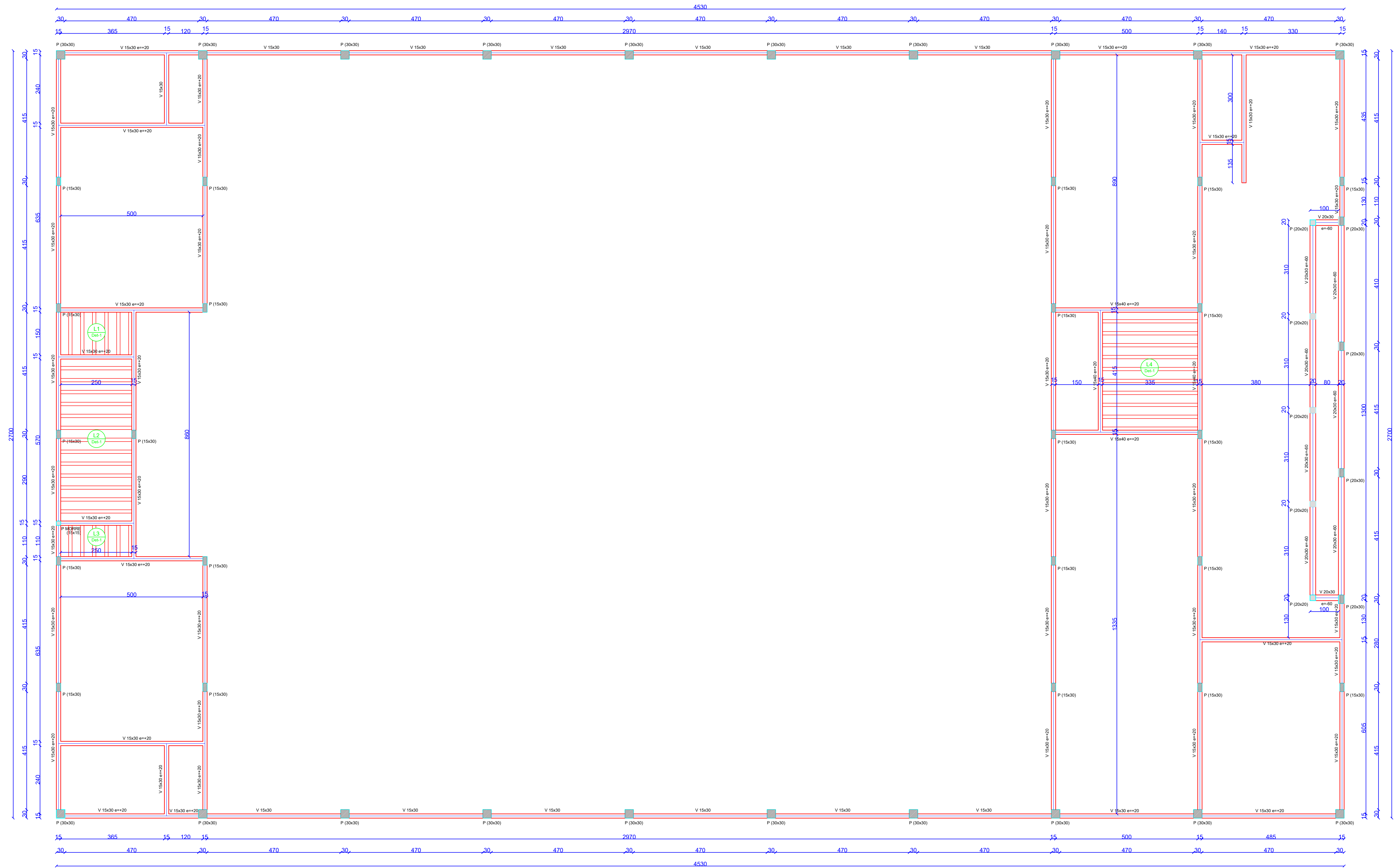
PLANTA DE FORMA DO PAV. INTERMEDIÁRIO (NÍVEL 285)
