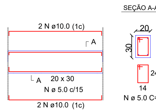
VIGAS (20X30)
