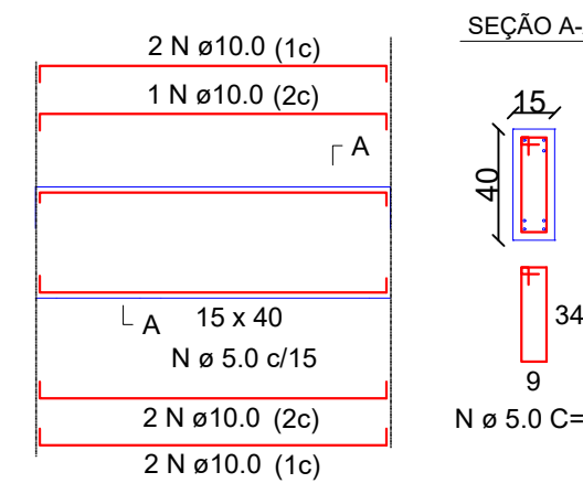
VIGAS (15X40) - CAIXA D'ÁGUA
